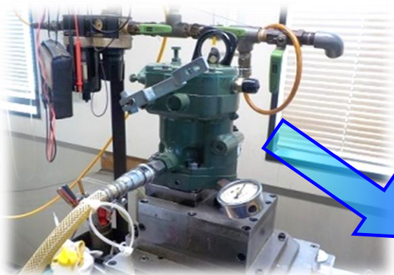
ガバナ単体による整備・ベンチテスト ガバナタイプ：Woodward PSG
