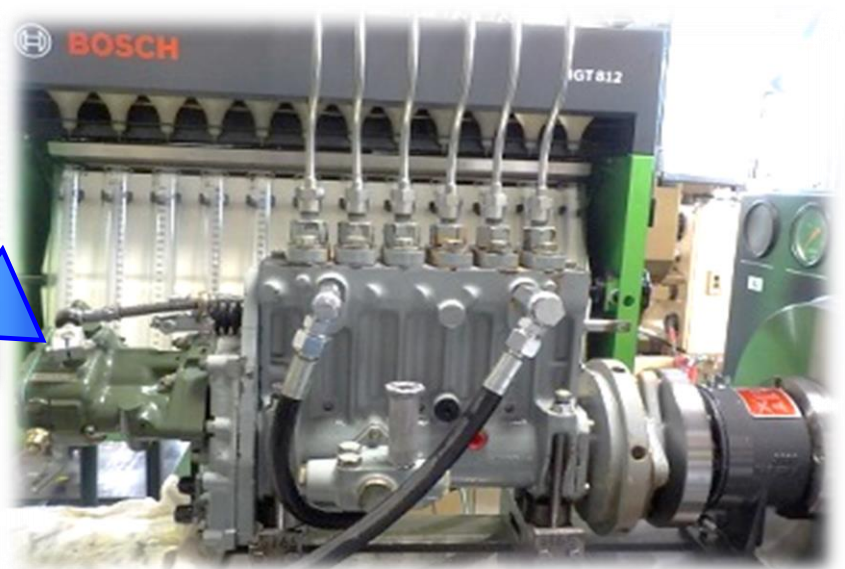
ガバナと燃料ポンプを接続した総合的なベンチテスト 燃料ポンプタイプ：PS-6
